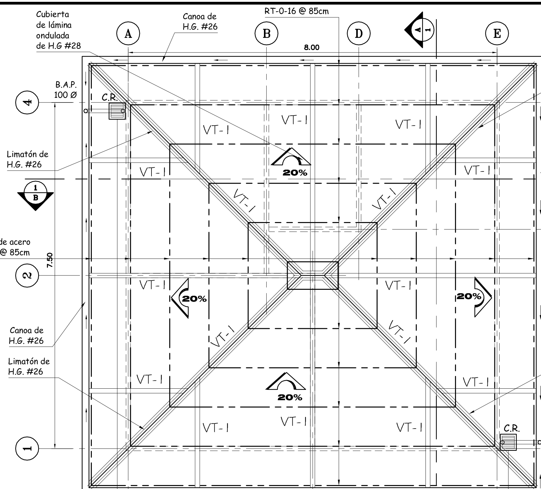
PLANTA DE TECHOS Y PLUVIALES. ESC 1:50
