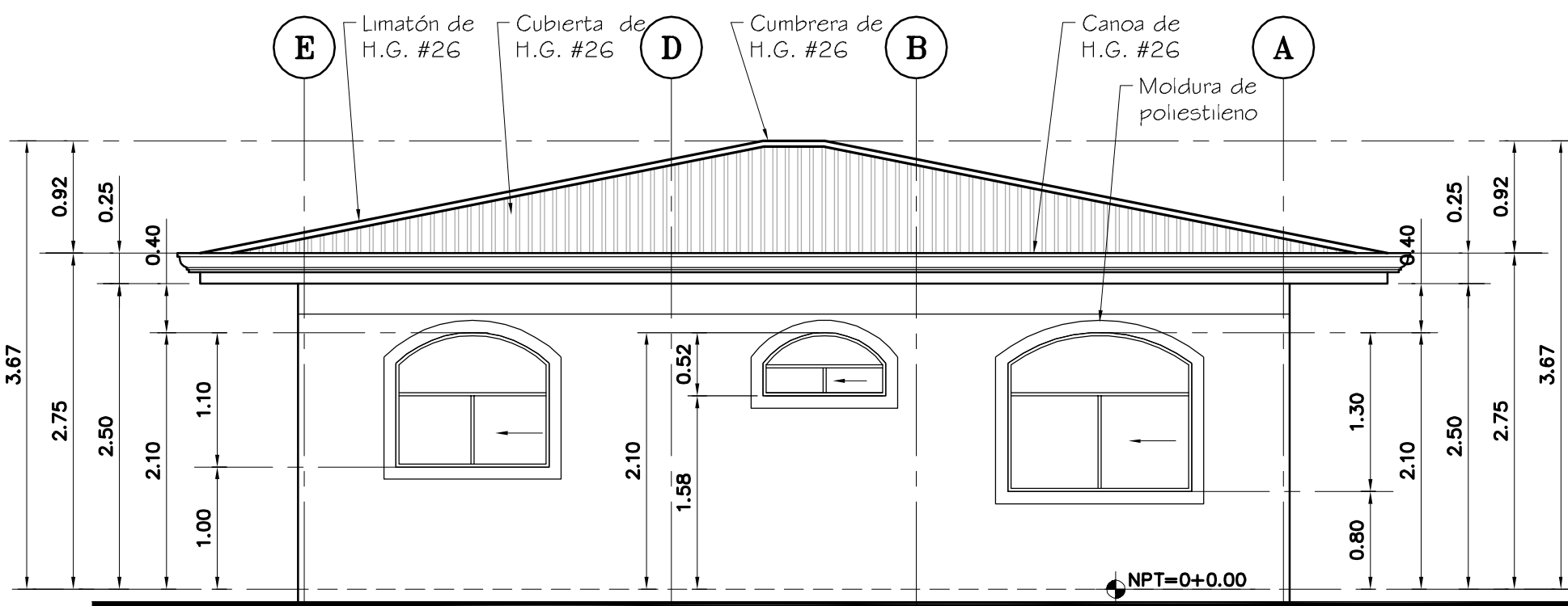
ELEVACION POSTERIOR. ESC 1:50
