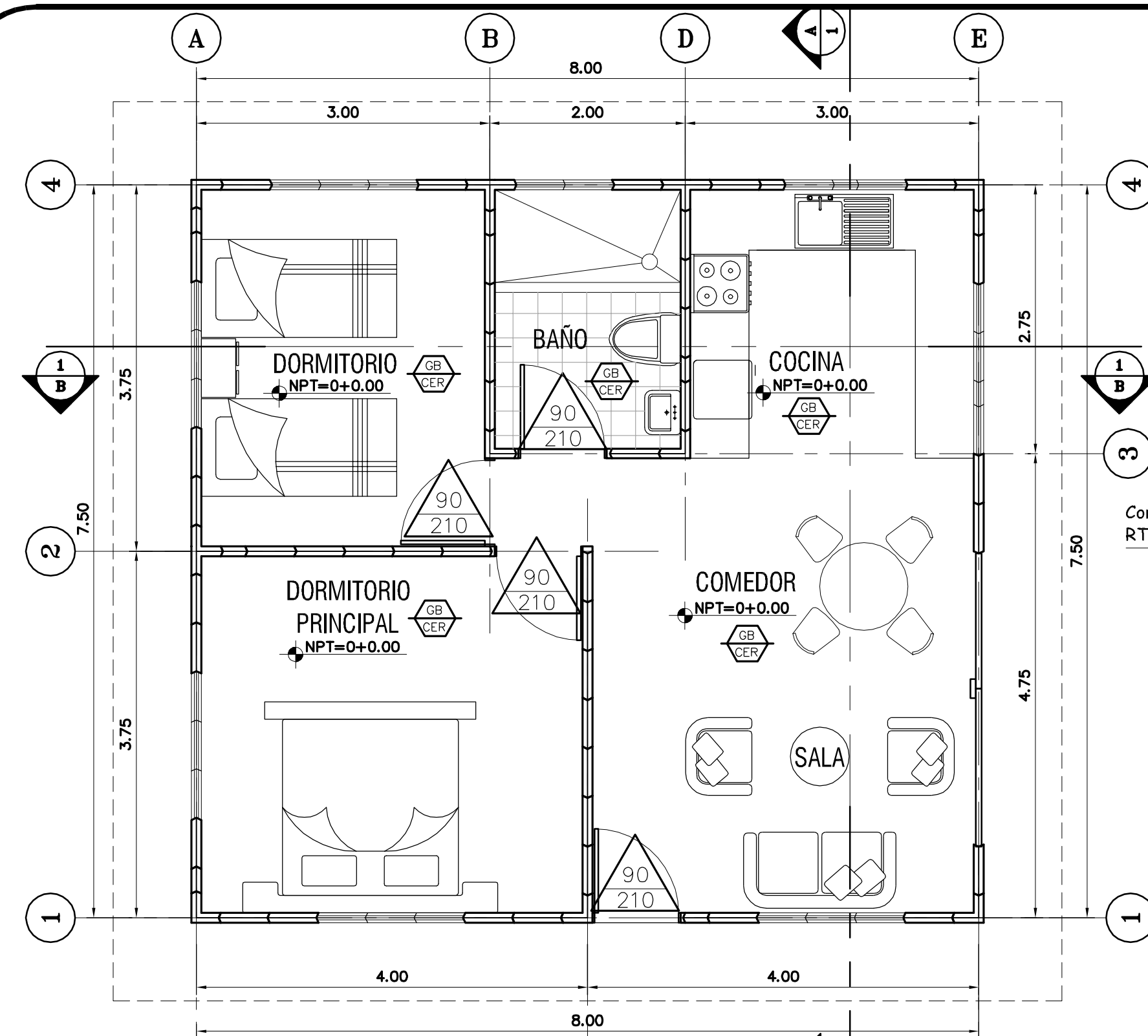
PLANTA DE DISTRIBUCION ARQUITECTONICA ESC 1:50
