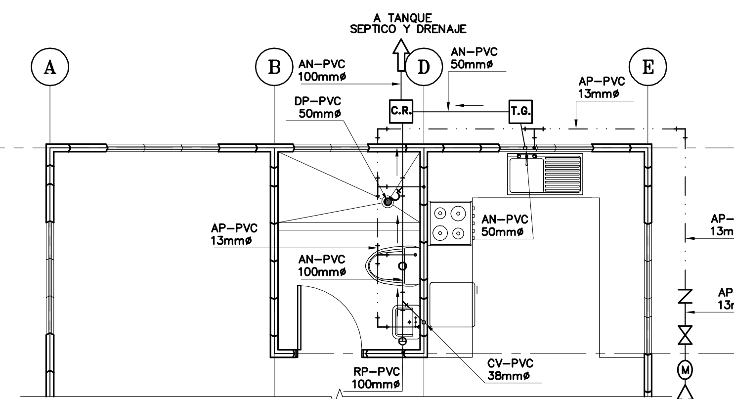
PLANTA DE INSTALACION MECANICA. ESC 1:50
