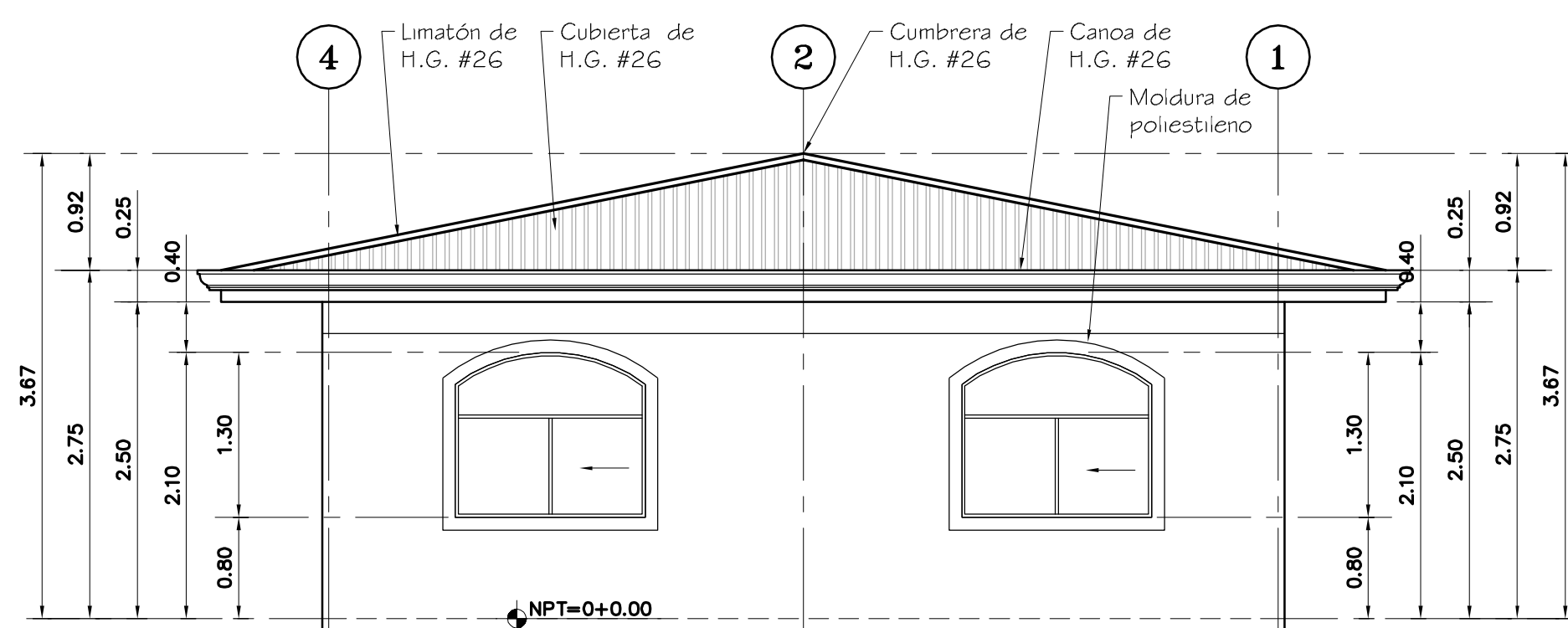
ELEVACION LATERAL IZQUIERDA. ESC 1:50
