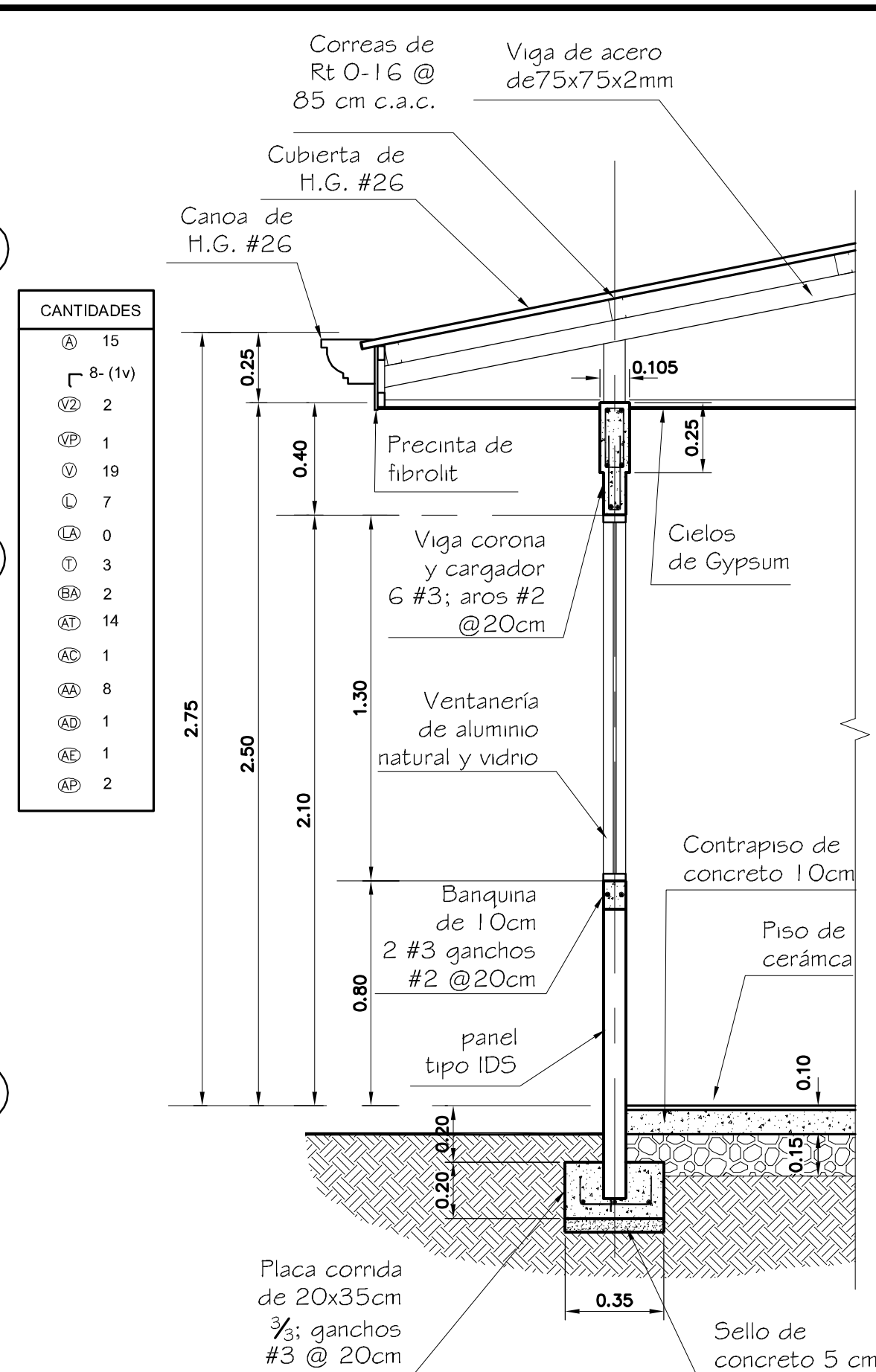
SECCION TIPICA. ESC 1:20
