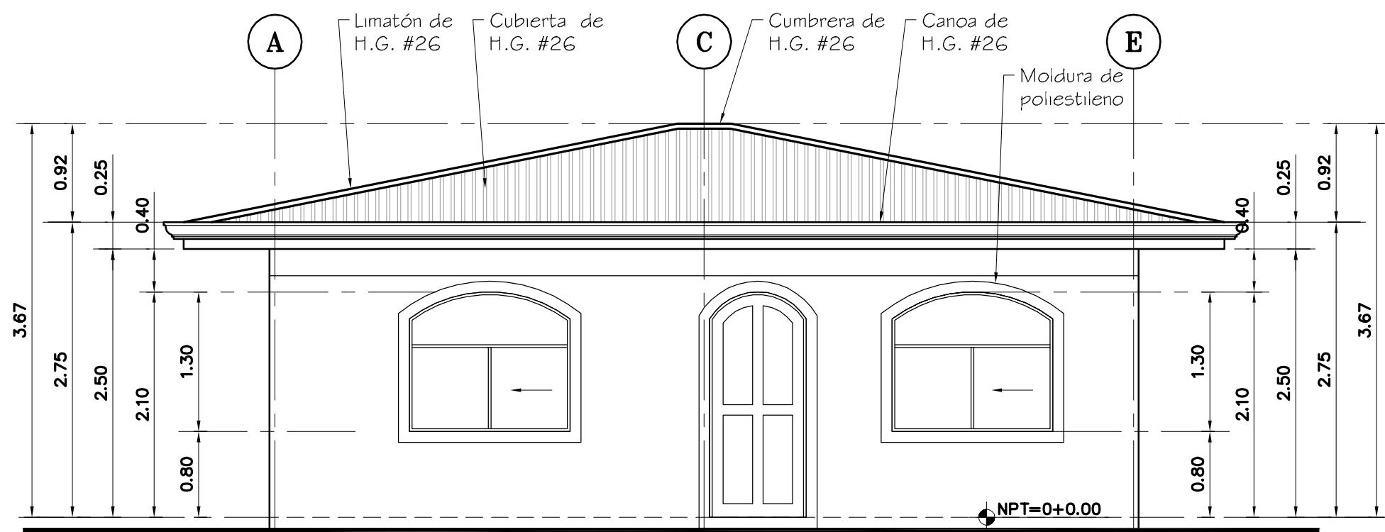
ELEVACION FRONTAL. ESC 1:50
