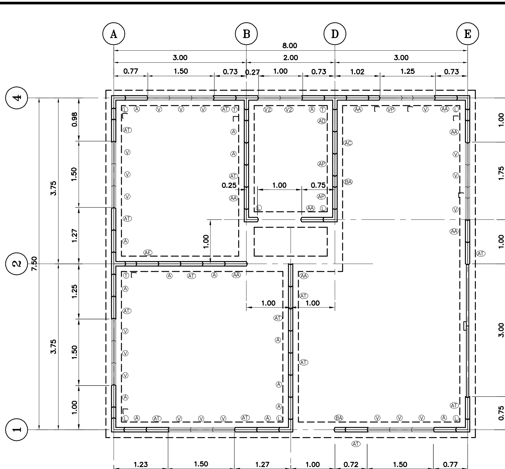
PLANTA DE FUNDACIONES Y ESTRUCTURAL ESC 1:50
