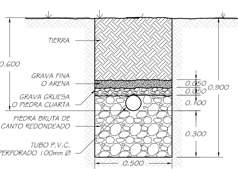
DET. DE DRENAJE ESC 1:15
