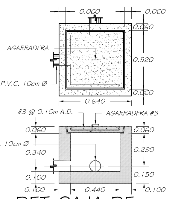
DET. CAJA DE REGISTRO ESC 1:20
