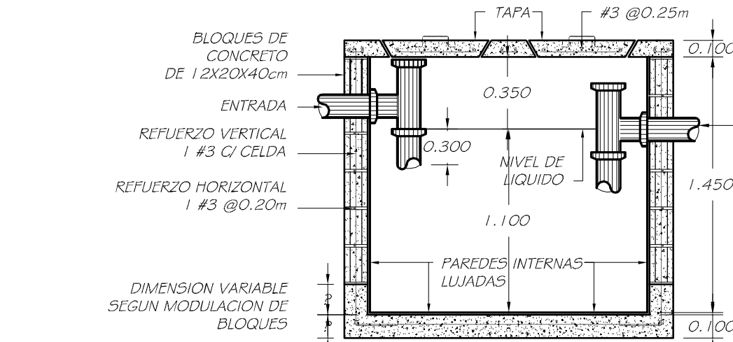
DET. DE TANQUE SEPTICO SIN ESCALA
