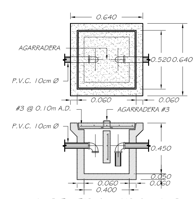
DET. TRAMPA DE GRASA ESC 1:20
