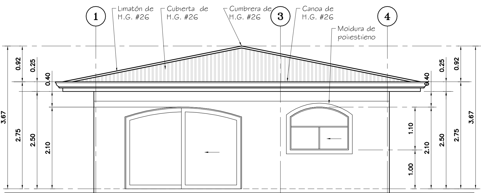
ELEVACION LATERAL DERECHA. ESC 1:50
